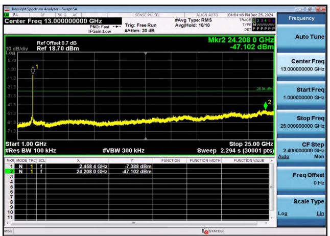
1GHz-25GHz
