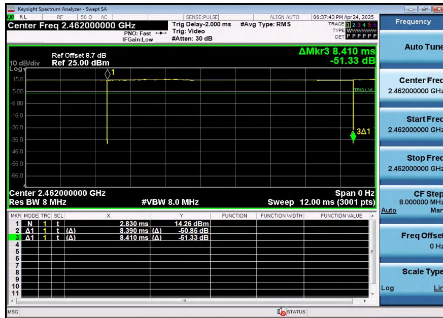
Ant1
