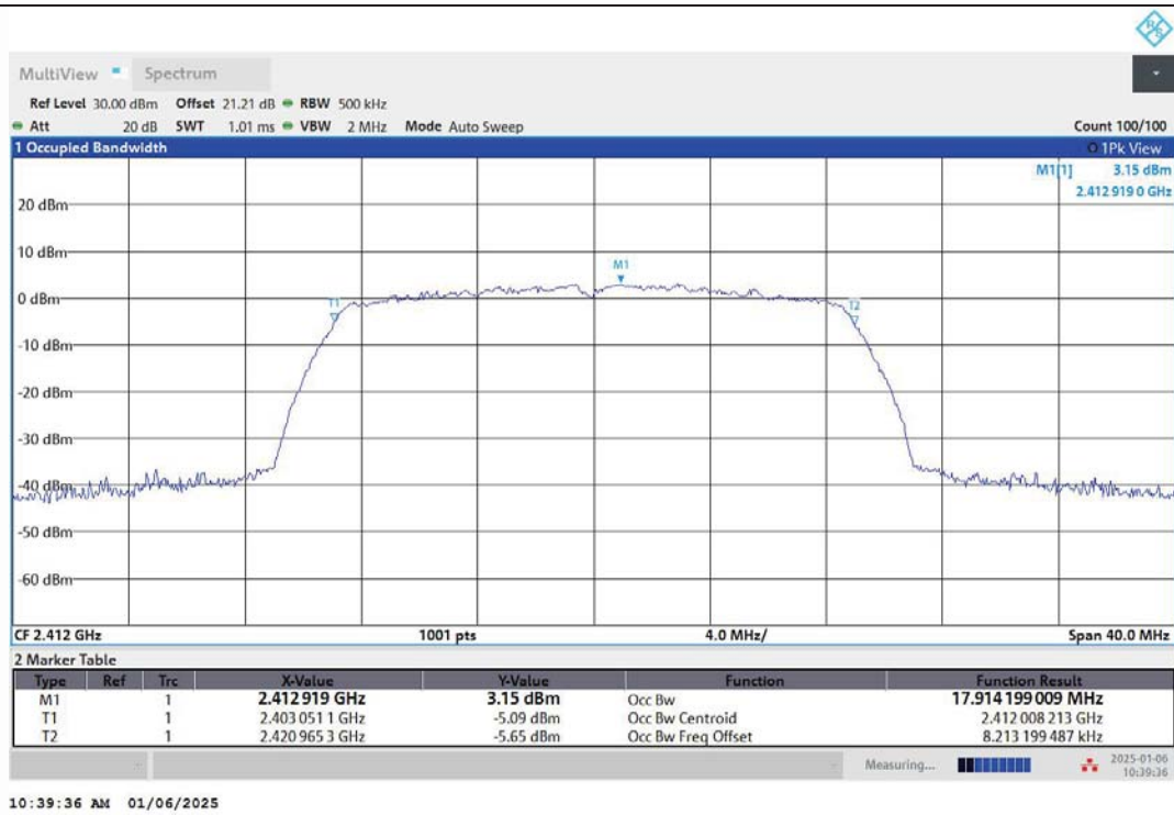
11N20MIMO-Ant1-2412
