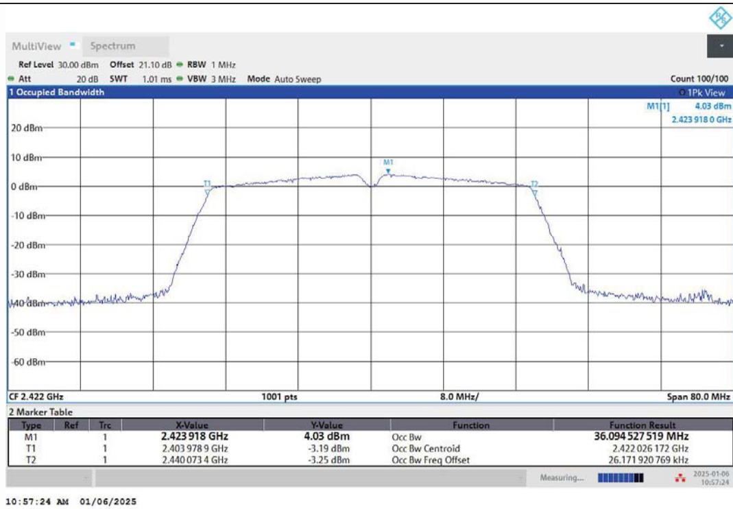
11N40MIMO-Ant1-2422
