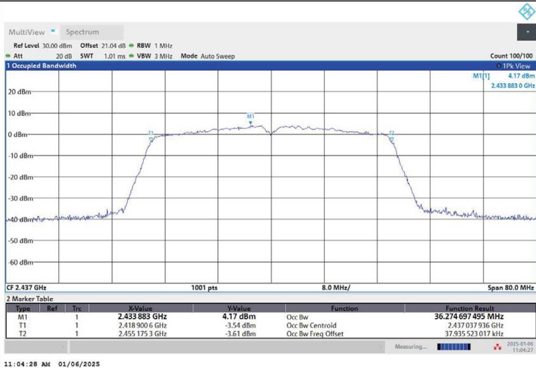
11N40MIMO-Ant2-2437
