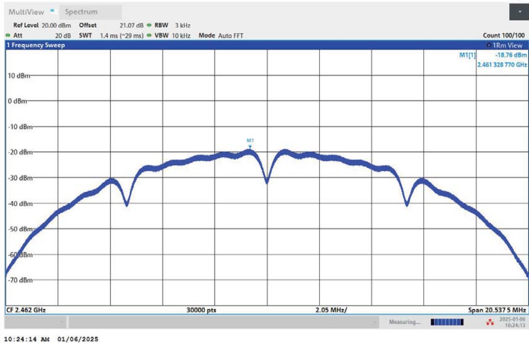
11B-Ant2-2462-PASS
