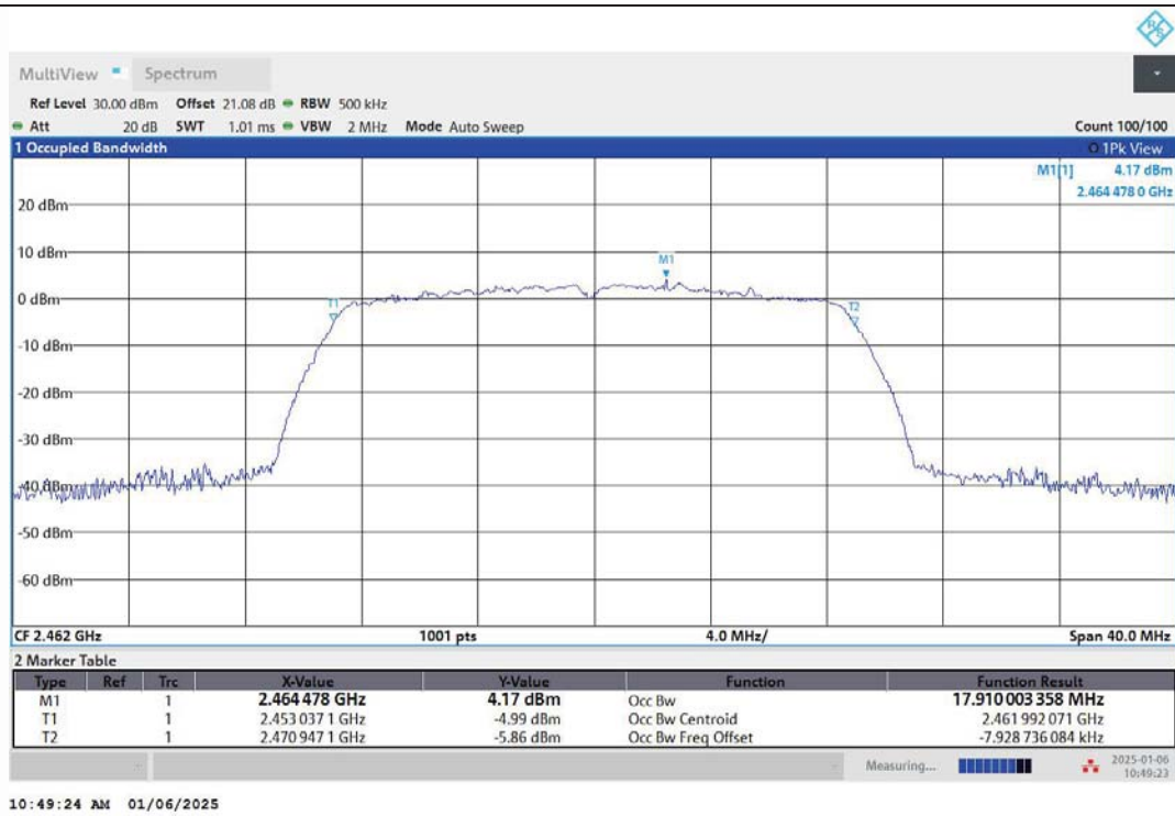
11N20MIMO-Ant1-2462
