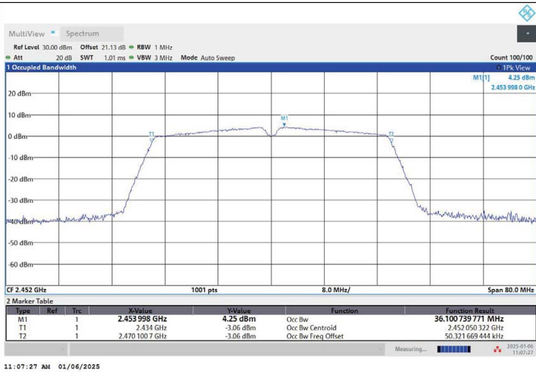
11N40MIMO-Ant1-2452
