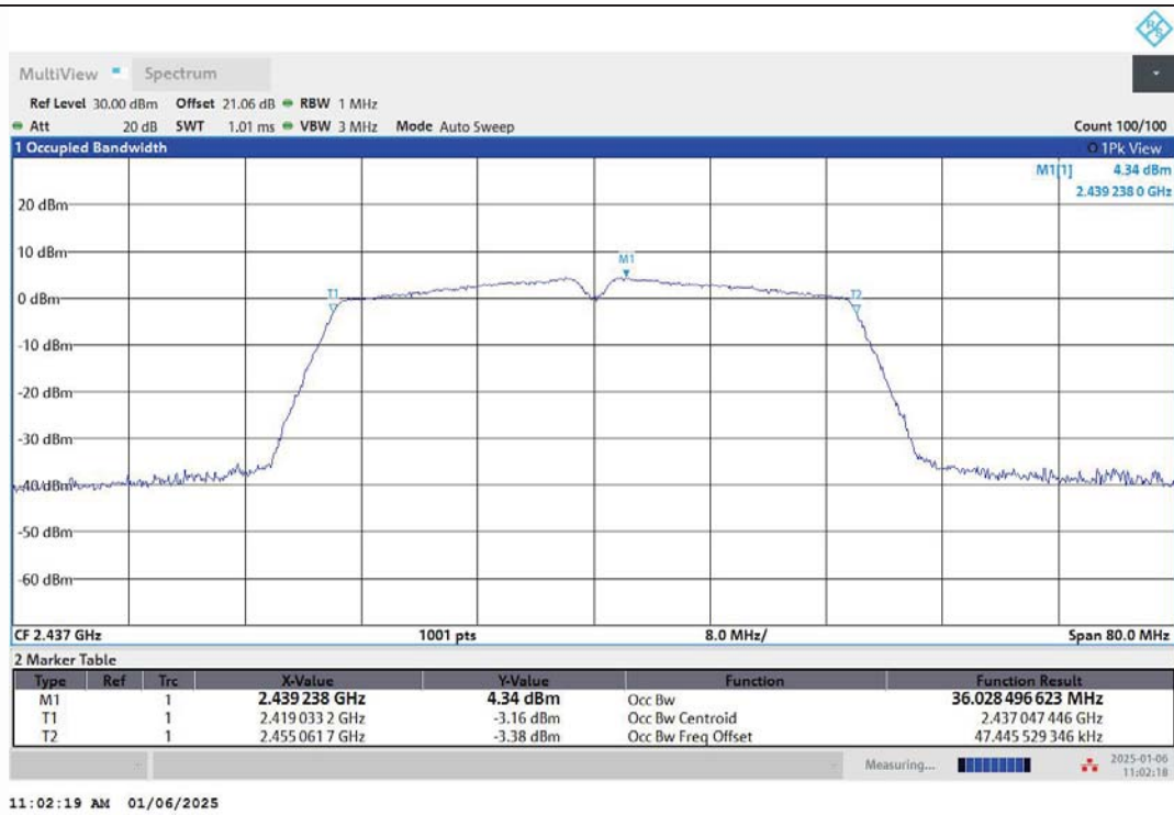
11N40MIMO-Ant1-2437
