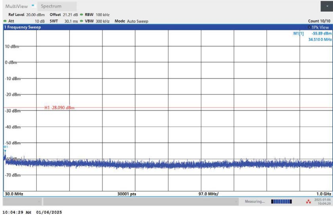
11G-Ant1-2412-30~1000-PASS
