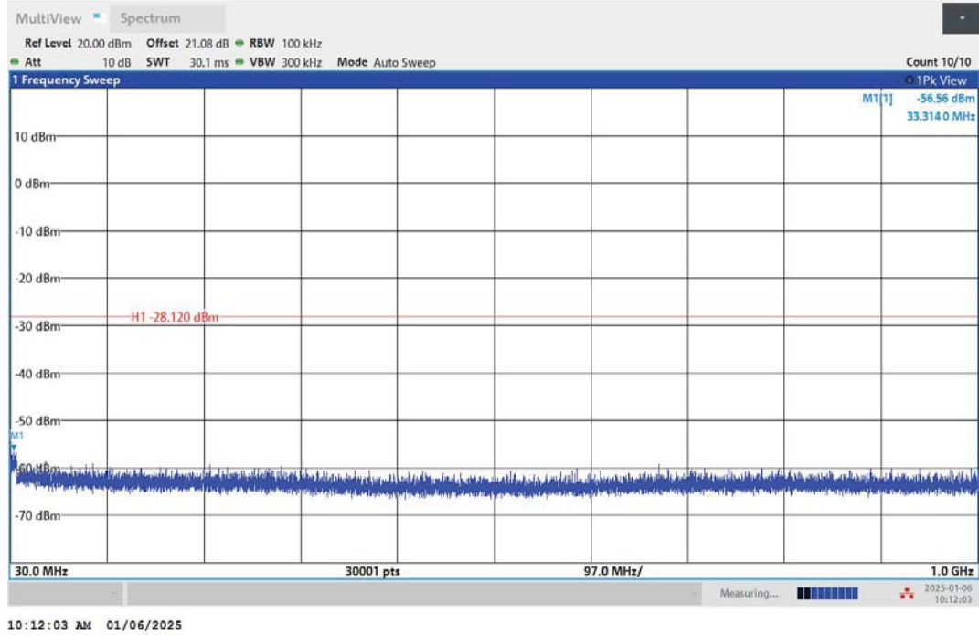
11G-Ant1-2462-30~1000-PASS
