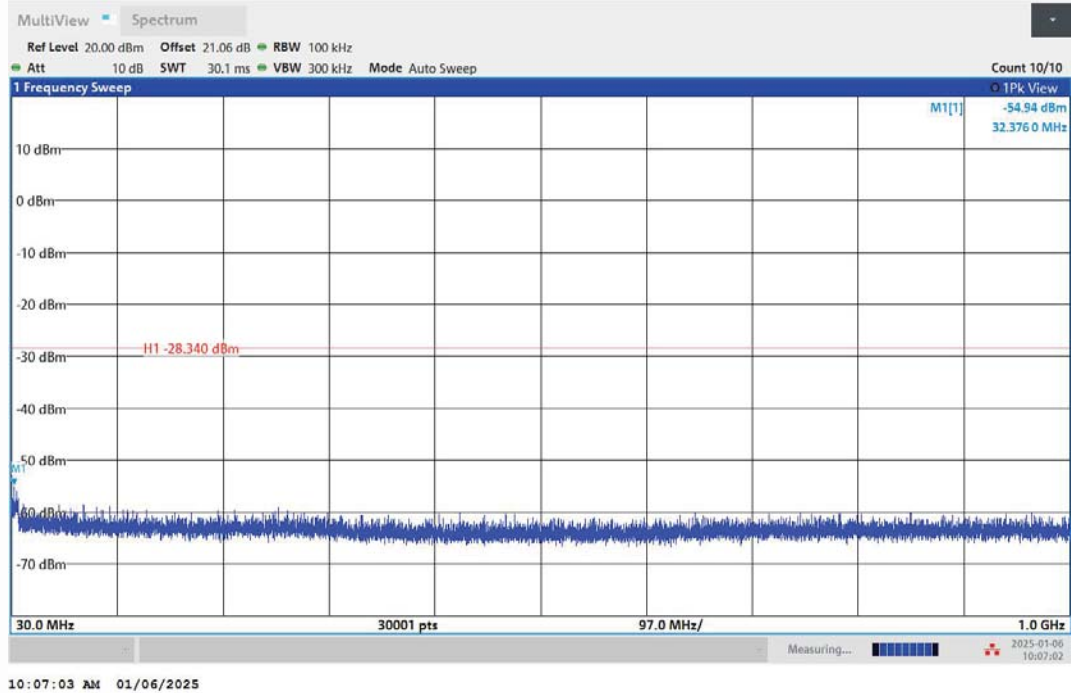
11G-Ant1-2437-30~1000-PASS
