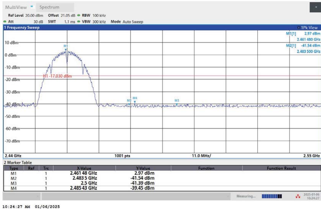
11B-Ant2-2462-PASS
