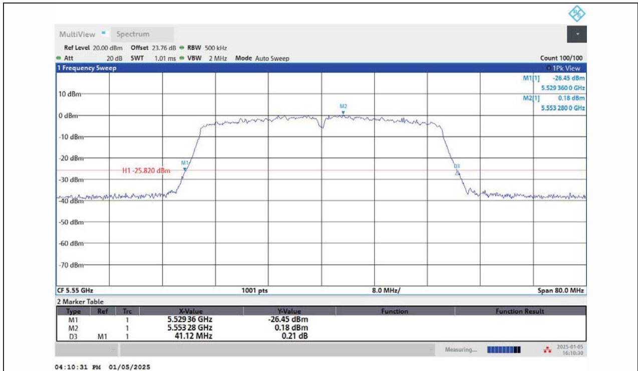
11N40MIMO-Ant1-5550
