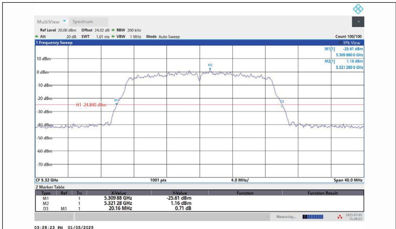
11N20MIMO-Ant1-5320
