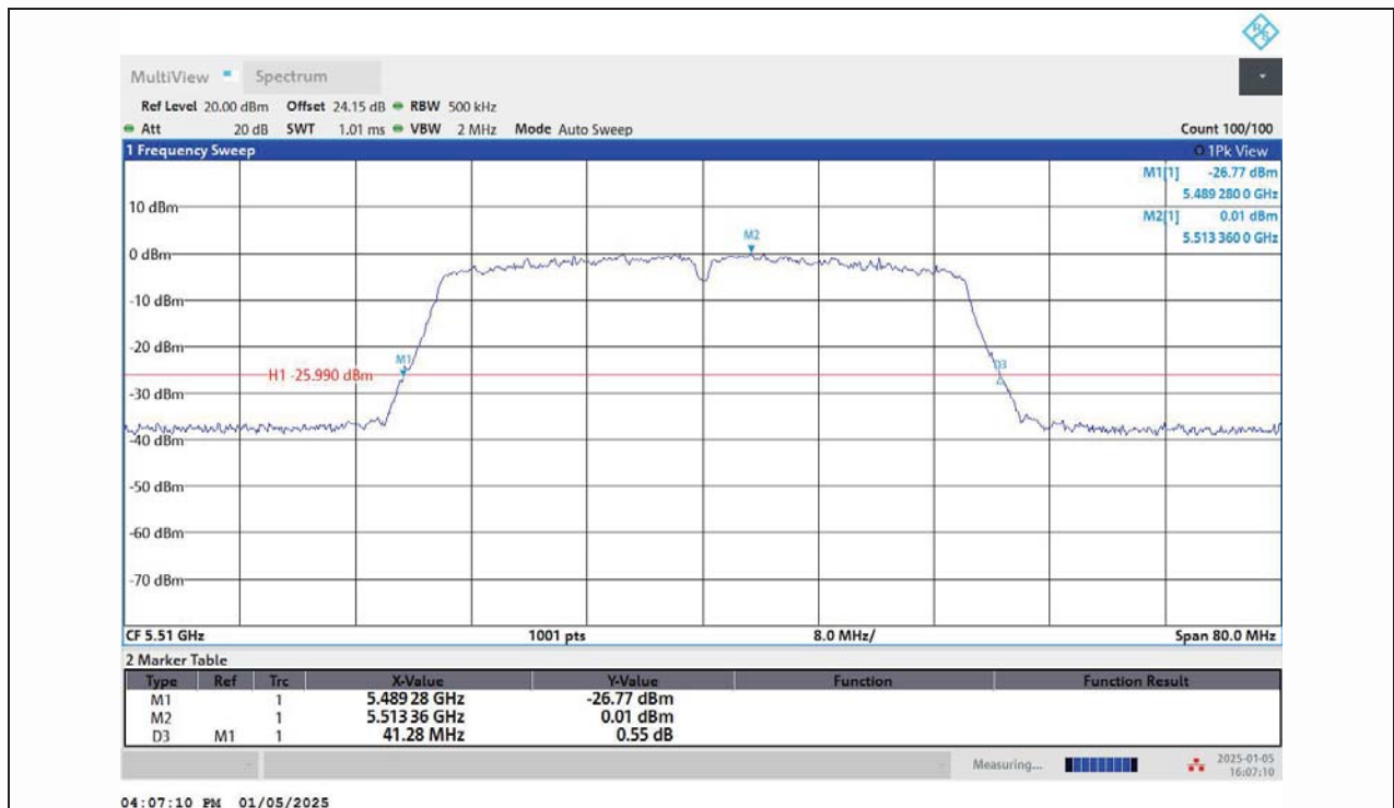
11N40MIMO-Ant1-5510
