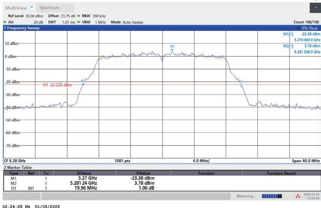
11A-Ant1-5280
