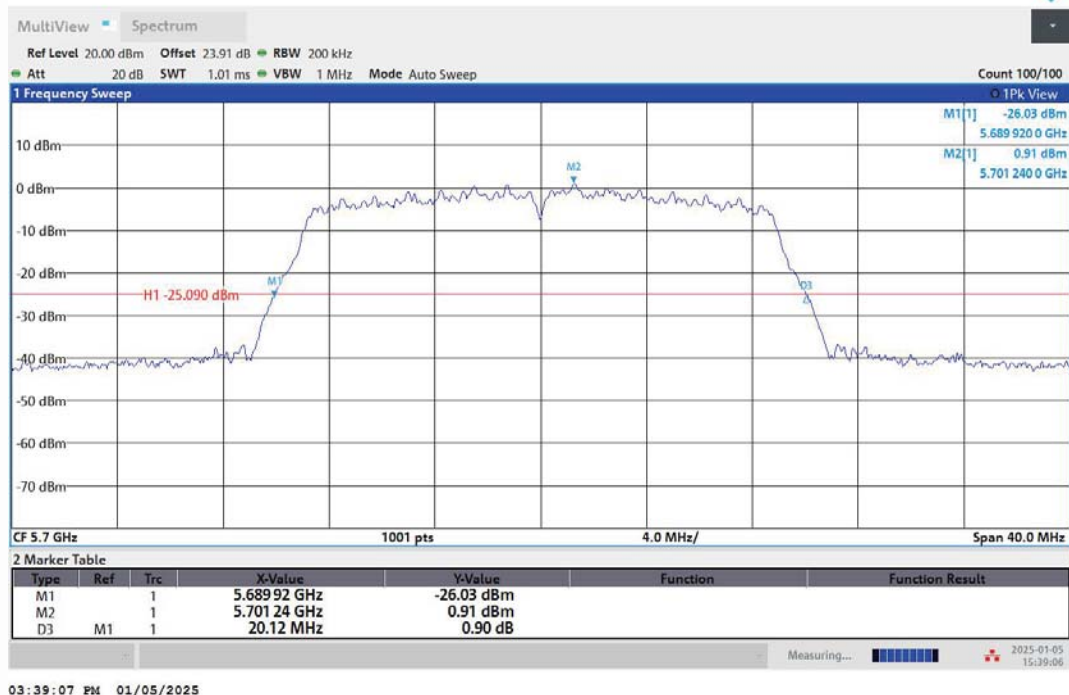
11N20MIMO-Ant1-5700
