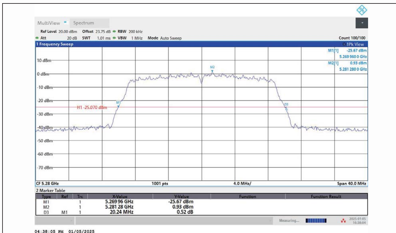
11AC20MIMO-Ant1-5280
