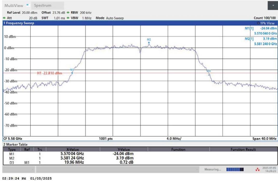
11A-Ant1-5580
