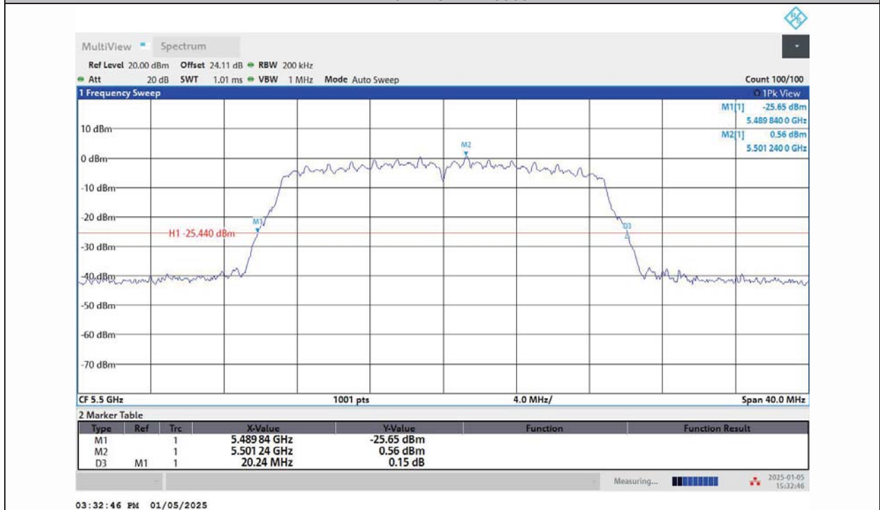
11N20MIMO-Ant2-5500
