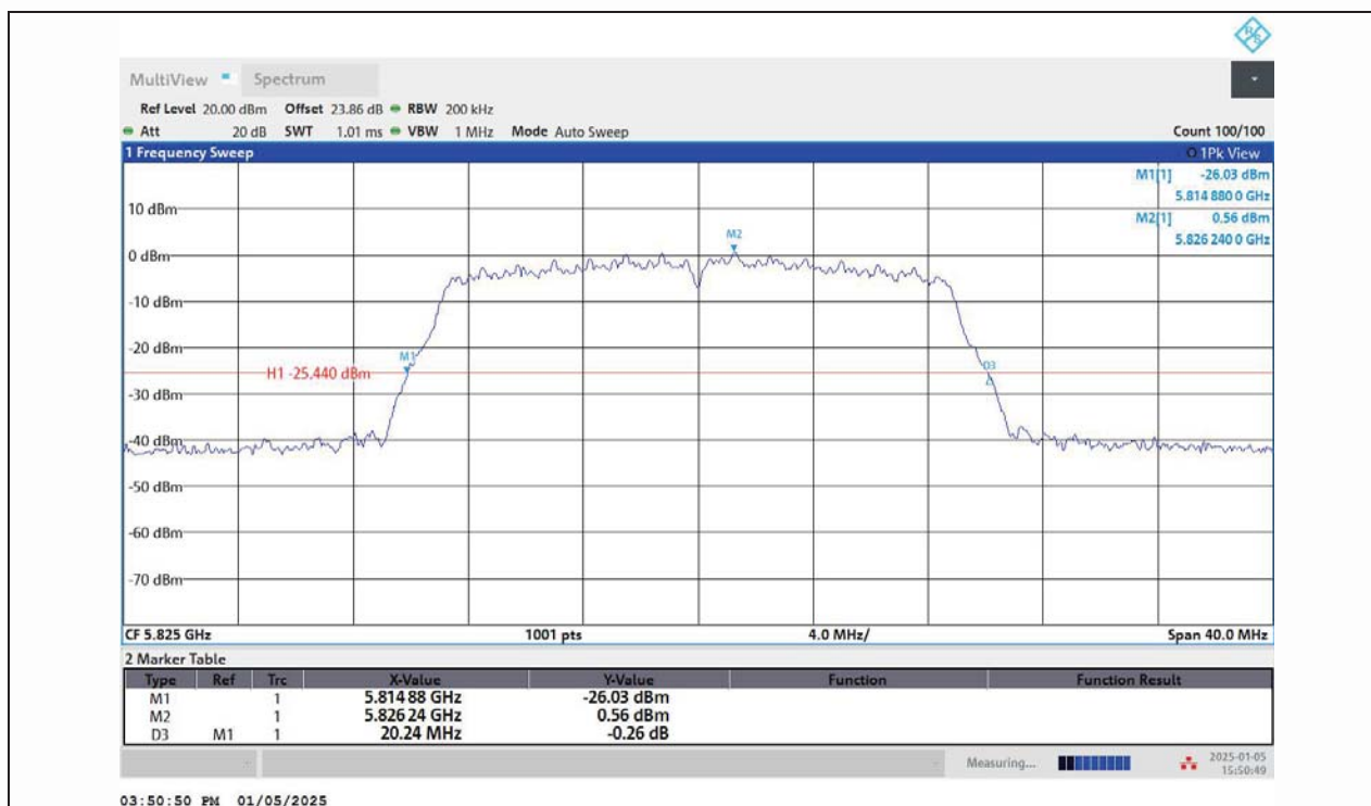
11N20MIMO-Ant1-5825
