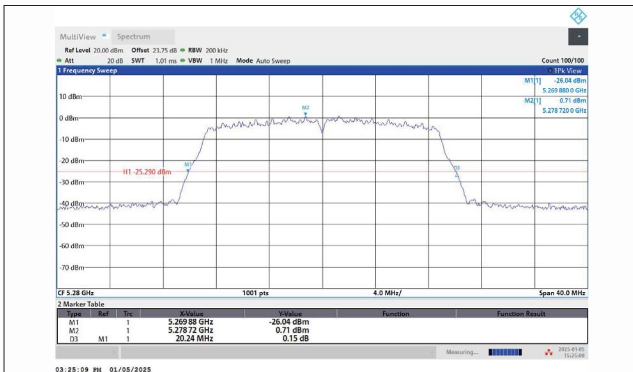
11N20MIMO-Ant1-5280
