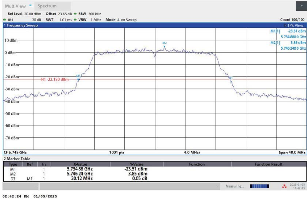
11A-Ant1-5745
