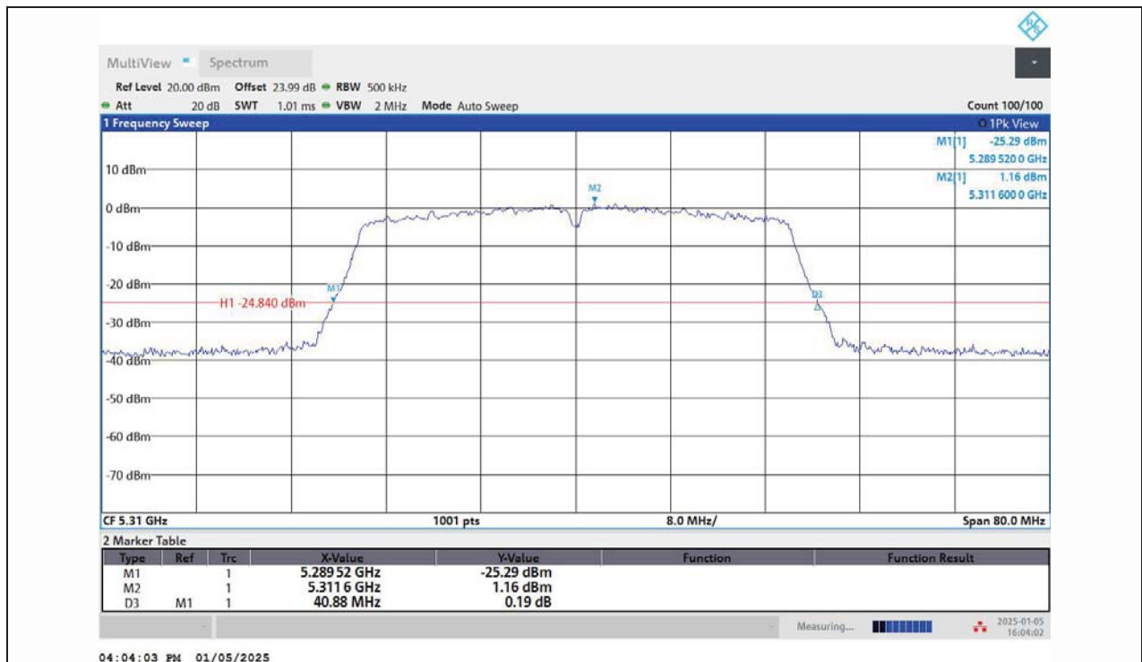
11N40MIMO-Ant1-5310
