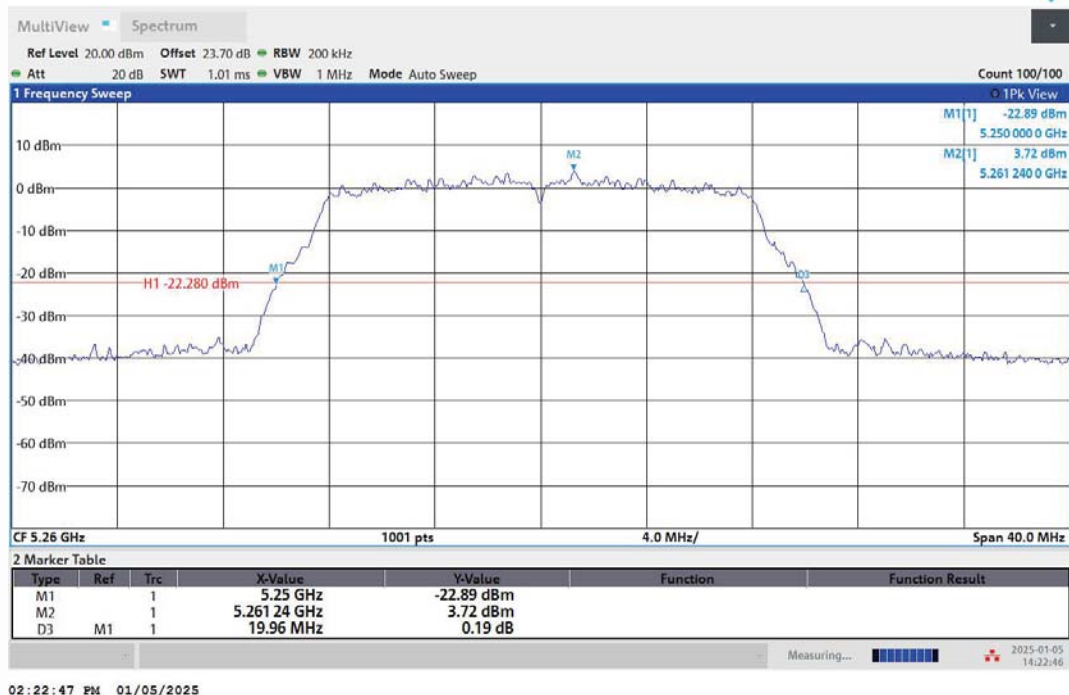
11A-Ant1-5260
