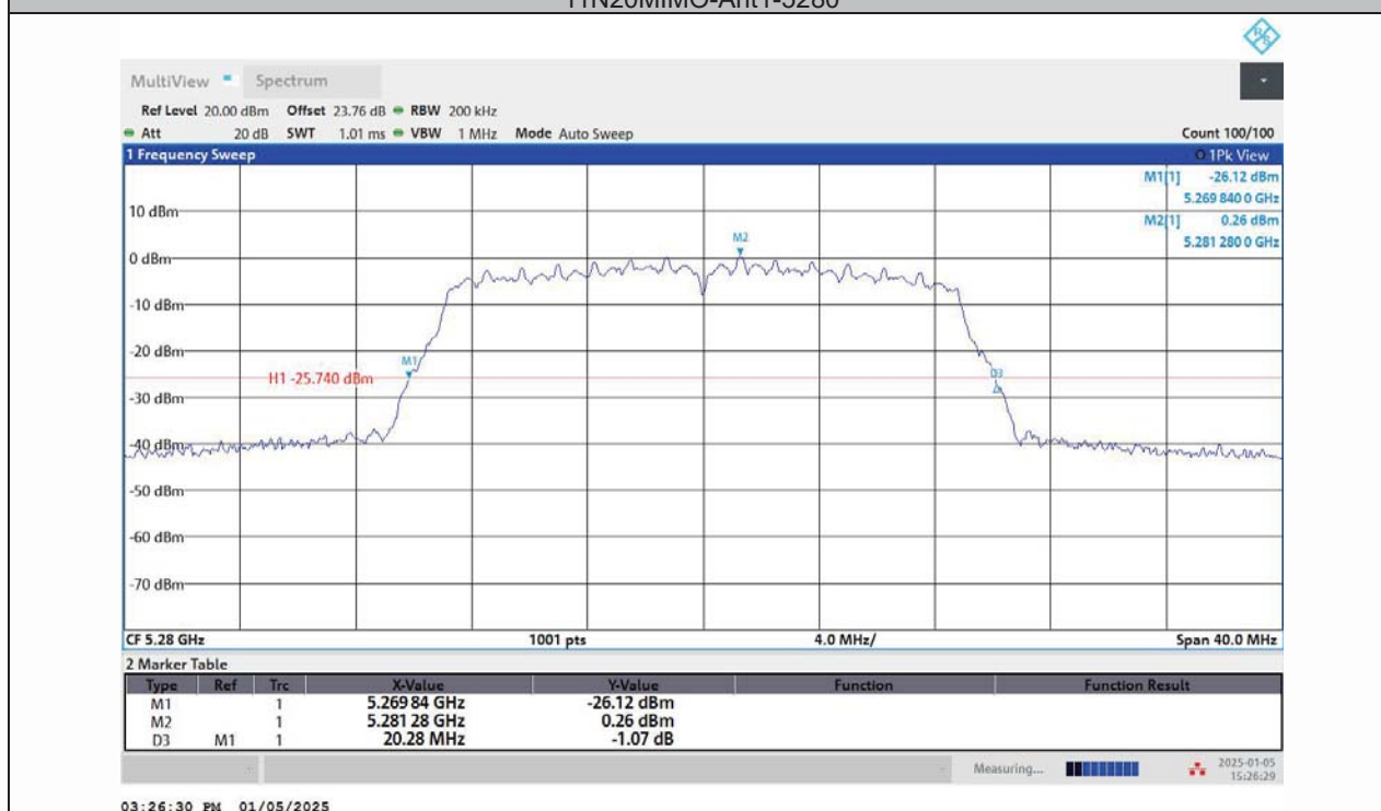
11N20MIMO-Ant2-5280
