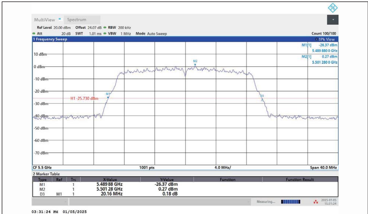
11N20MIMO-Ant1-5500
