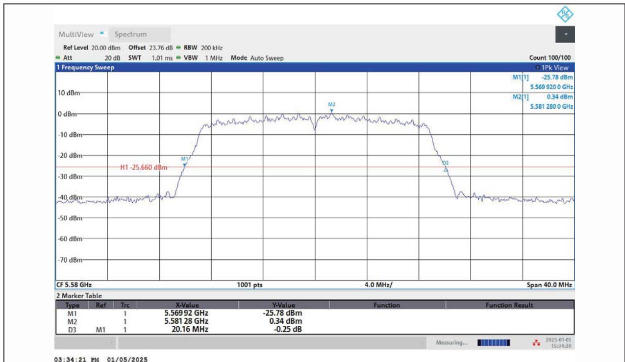
11N20MIMO-Ant1-5580
