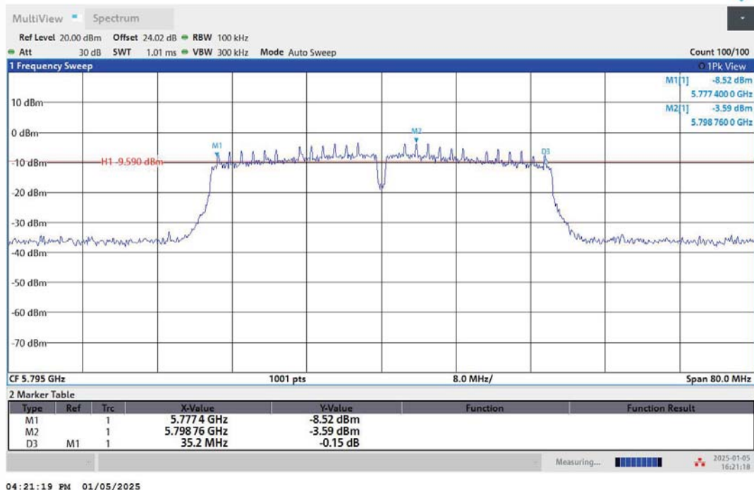
11N40MIMO-Ant1-5795-PASS
