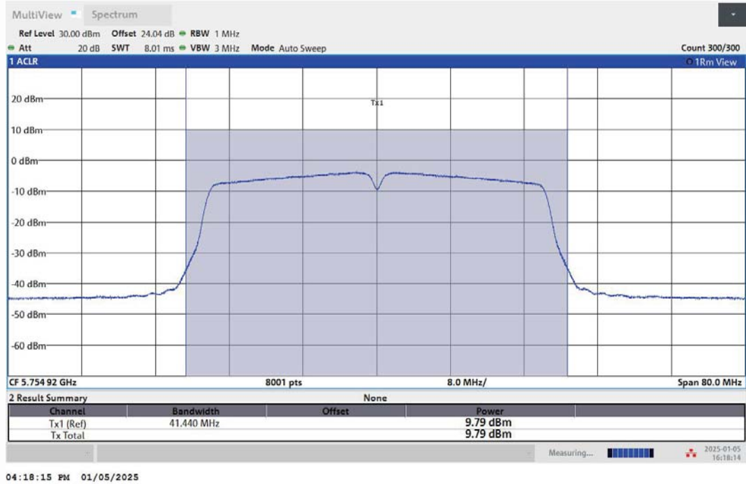
11N40MIMO-Ant1-5755-PASS
