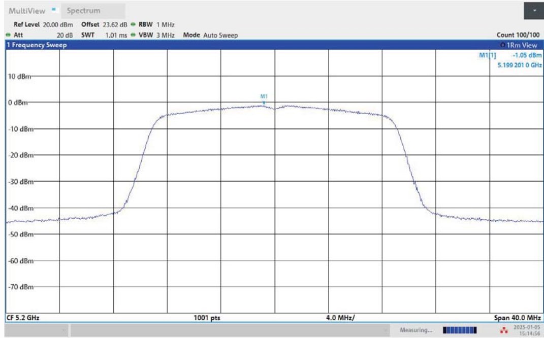
11N20MIMO-Ant1-5200-PASS
