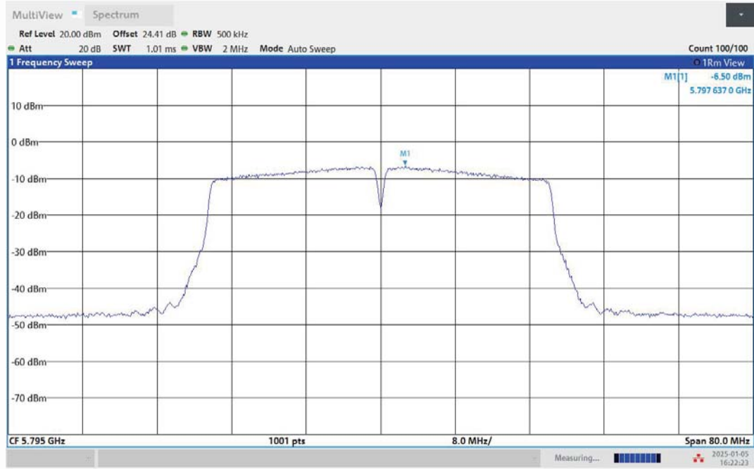
11N40MIMO-Ant1-5795-PASS
