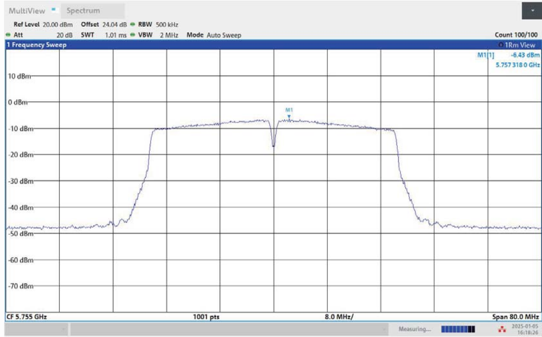
11N40MIMO-Ant1-5755-PASS
