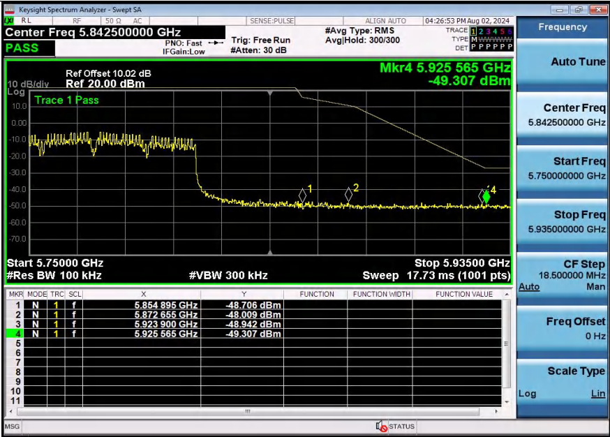
11AX80SISO-Ant2-5775-PASS
