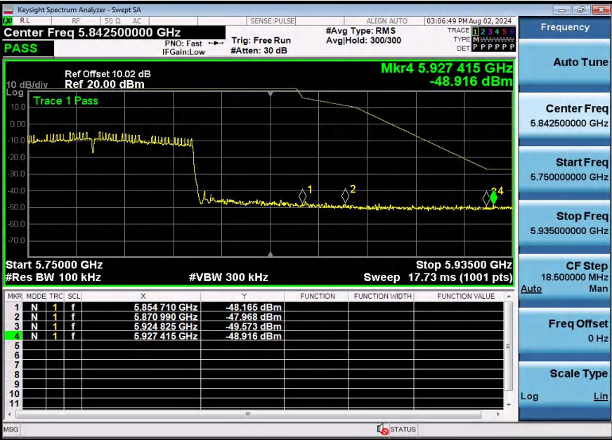
11AC80SISO-Ant2-5775-PASS
