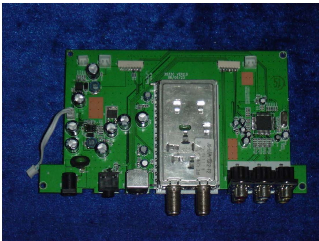
PCB Top
