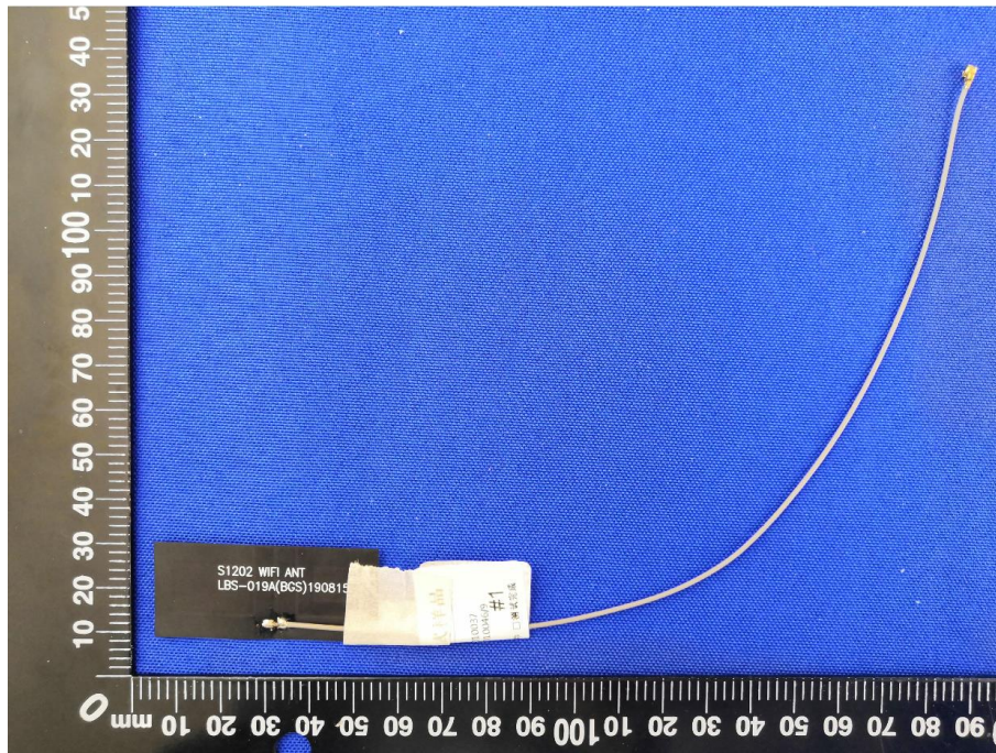
Antenna-SE-1202
