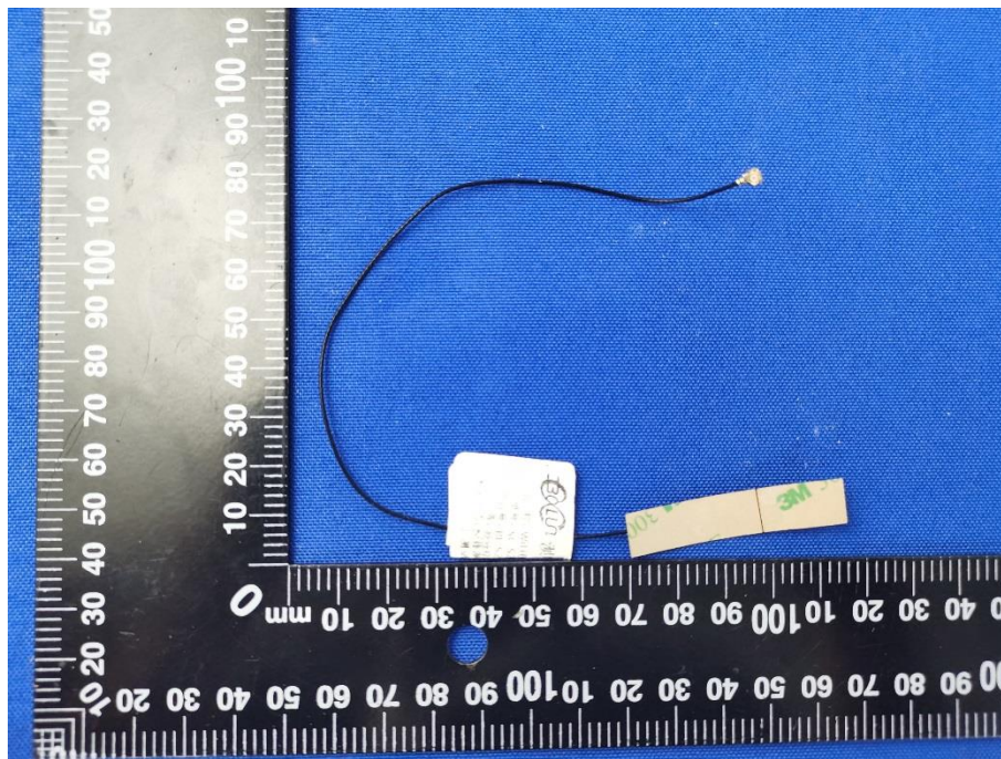
Antenna-i15/i15VET/i15A
