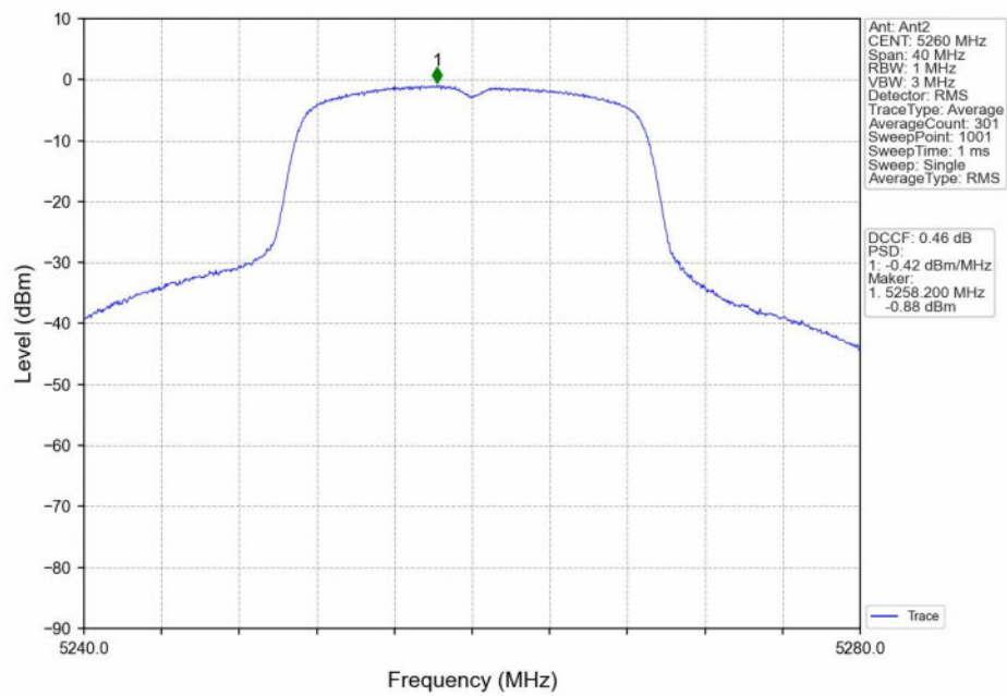
802.11n(HT20)_LCH_5260MHz_Ant2_NTNV
