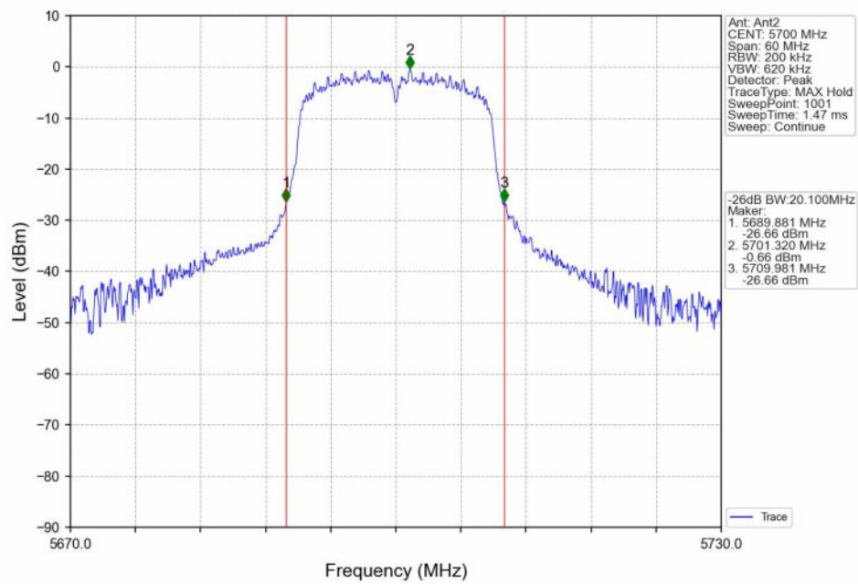
802.11n(HT20)_HCH_5700MHz_Ant2_NTNV
