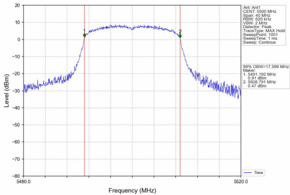
802.11ac(VHT20)_LCH_5500MHz_Ant1_NTNV
