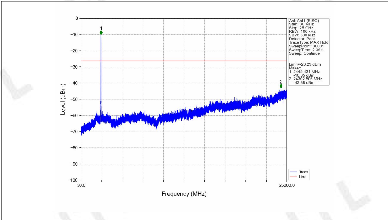
802.11n(HT40)_HCH_2452MHz_Ant1 (SISO)_NTNV
