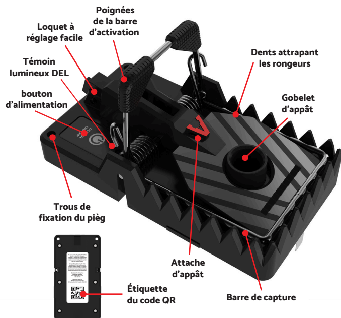
Modèle de piège à rats Victor® VLINK® : V430B
