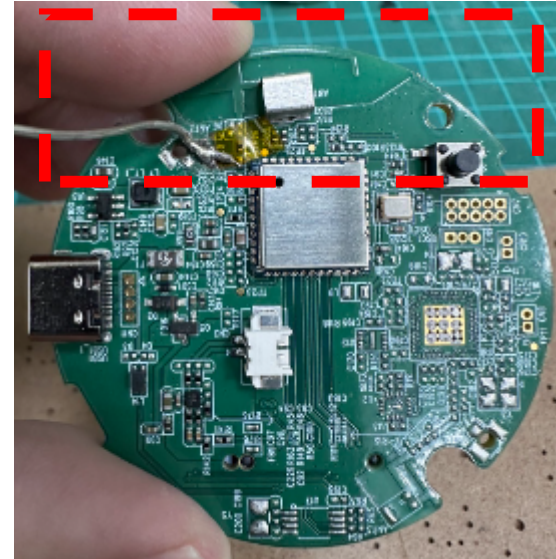
BQ0104S43001 2.4G/5G ANT
