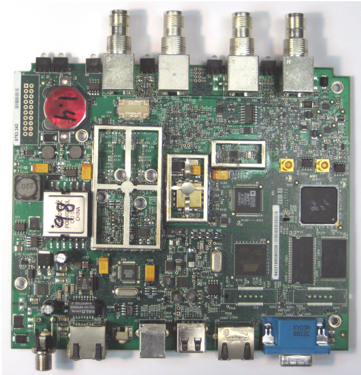
PCB Top
