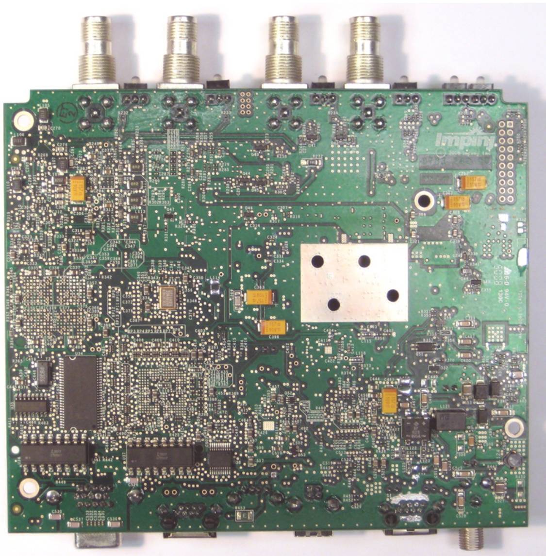
PCB Bottom
