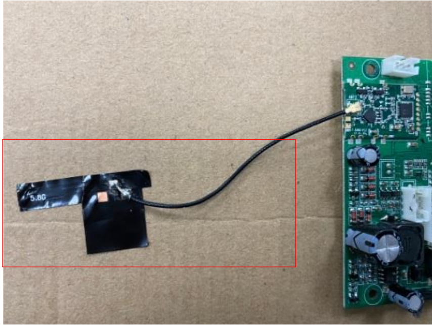
5.8G Antenna
