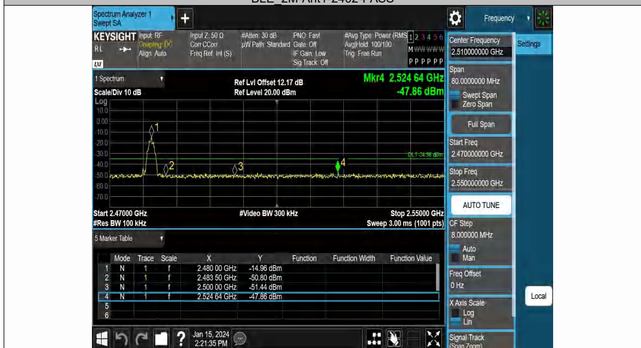
BLE 2M-Ant1-2480-PASS
