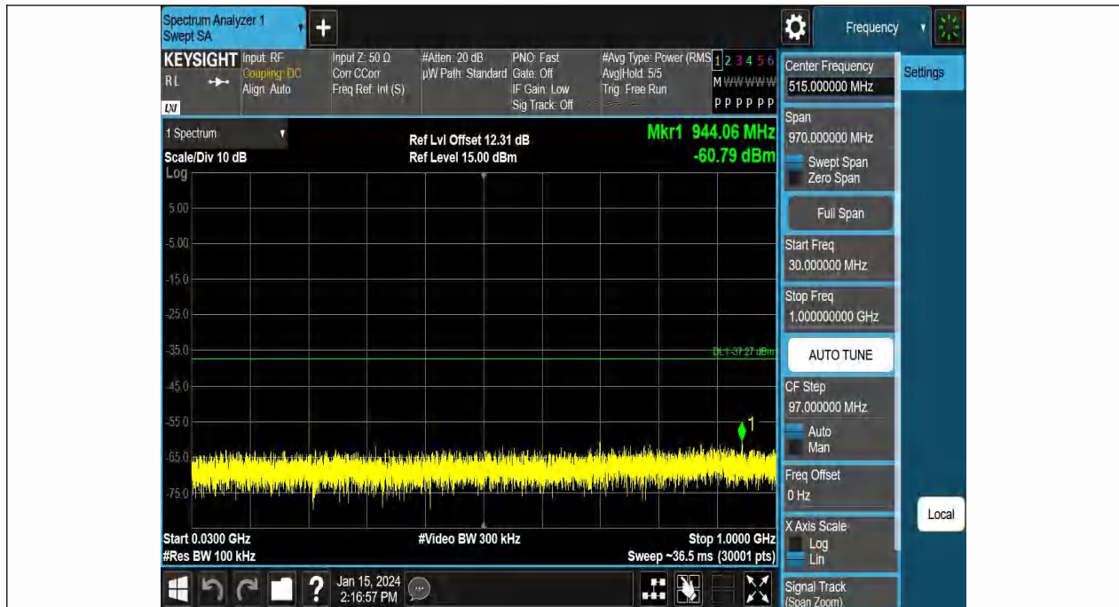
BLE_2M-Ant1-2402-30~1000-PASS
