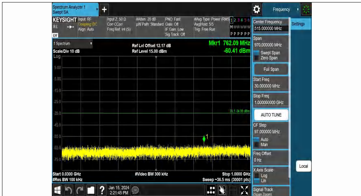
BLE_2M-Ant1-2480-30~1000-PASS
