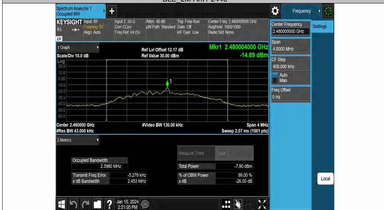
BLE_2M-Ant1-2480
