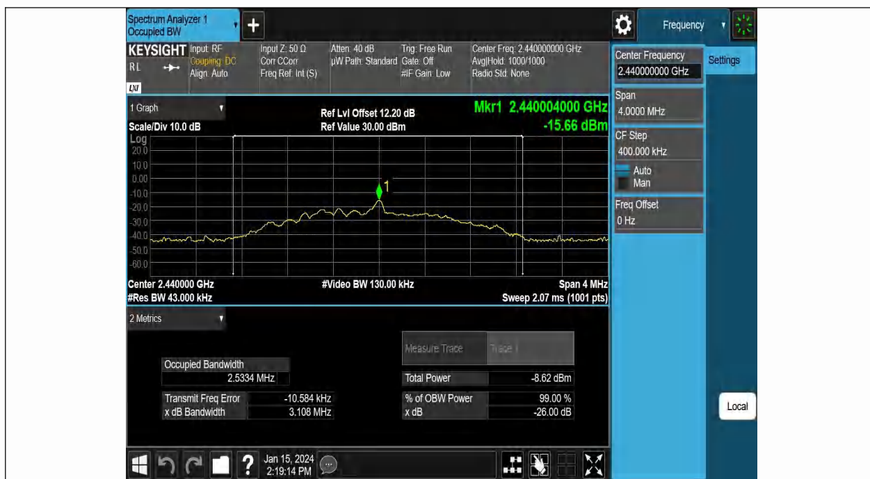
BLE_2M-Ant1-2440
