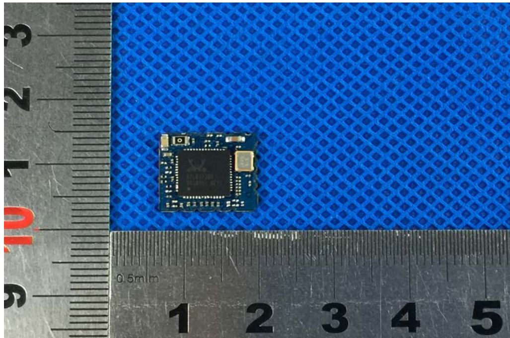
Photo 25 wifi/BT module
