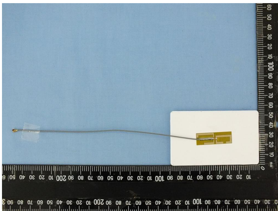
Antenna: MAF95310 Mini NanoBlade Flex
