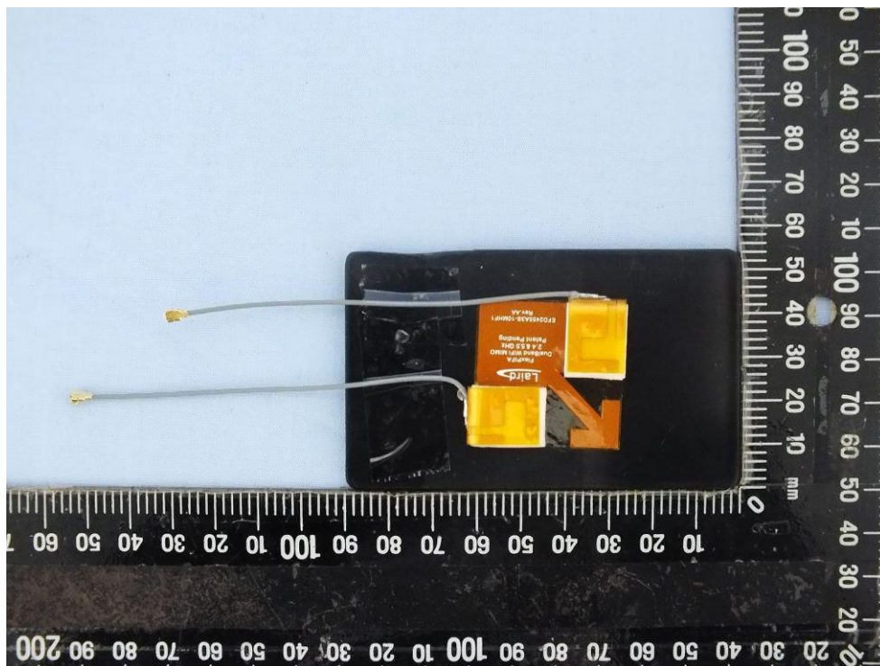
Antenna: MIMO FlexPIFA Antenna EFD2455A3S-10MHF1
