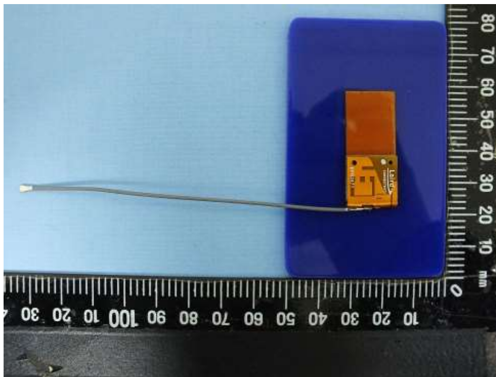
Ant.: EFB2471A3S-10MH4L
