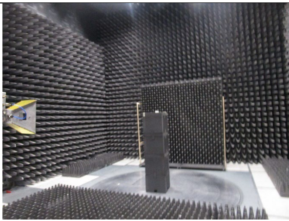
1-18 GHz
