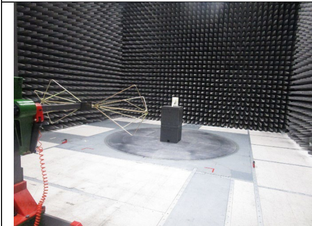
30-200 MHz
