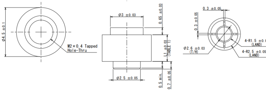
JAE SM3ZS067U310-NUT1-Rxxxx
