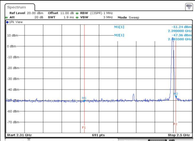
2480MHz - PK
