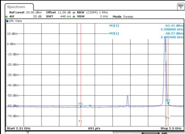
2480MHz - AV
