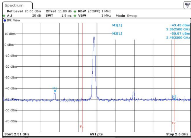
2440MHz - PK
