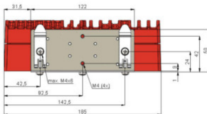
Fig. 2.8: L-bracket
