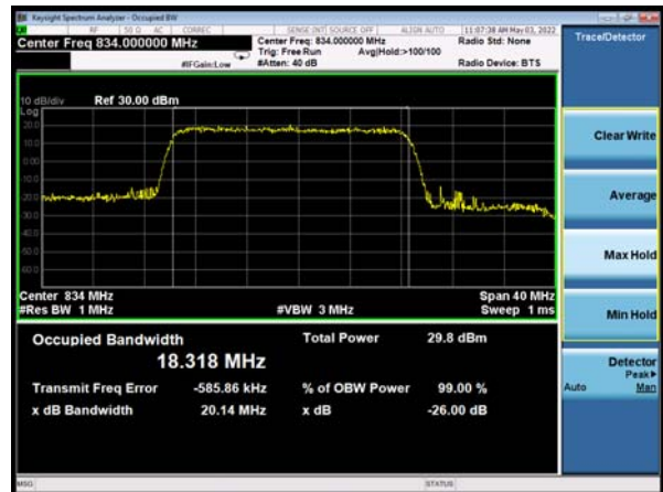
DC_66A-n5A 64QAM 20MHz CH-Middle
