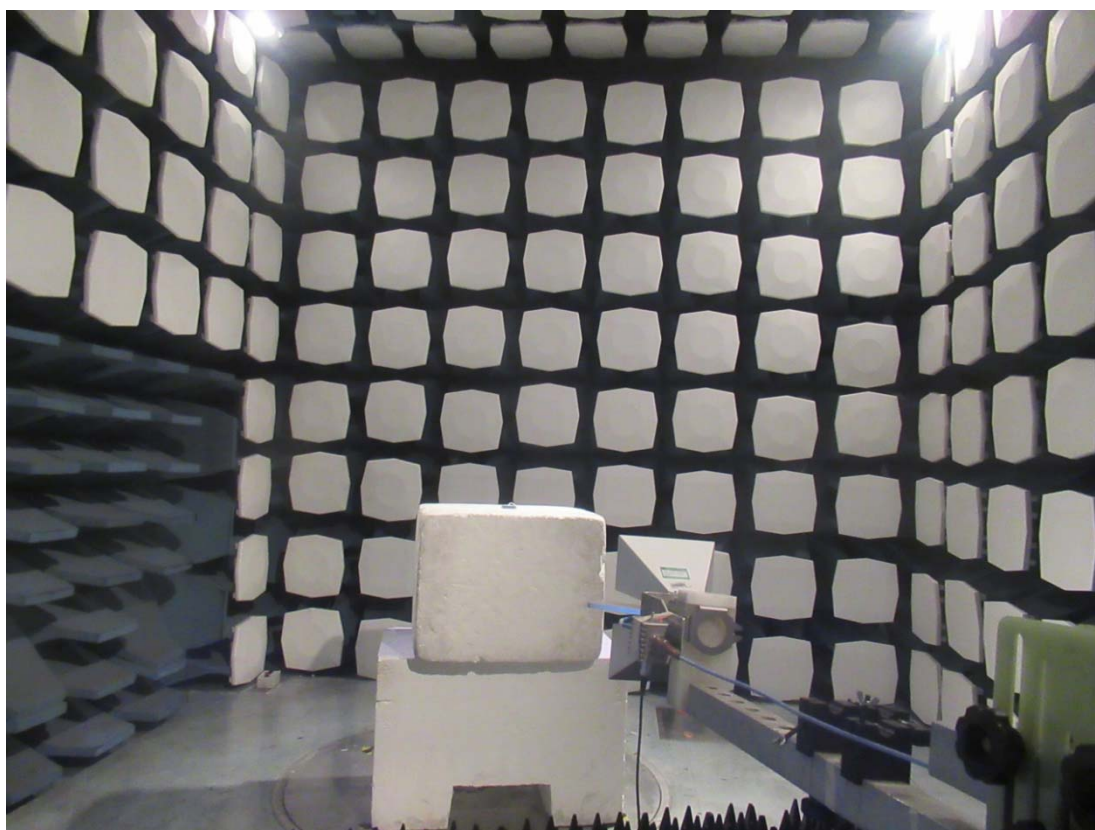
1GHz-18GHz
