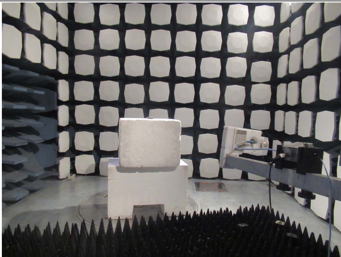
18GHz - 26.5GHz
