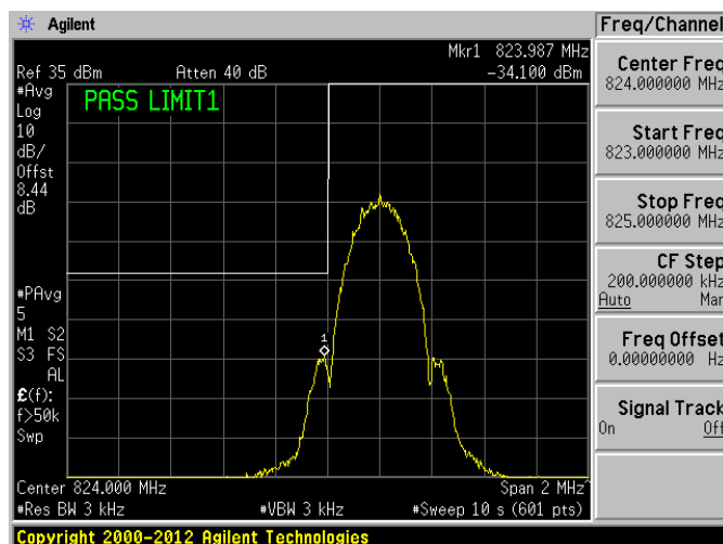
EGPRS 850 MHz LCH
