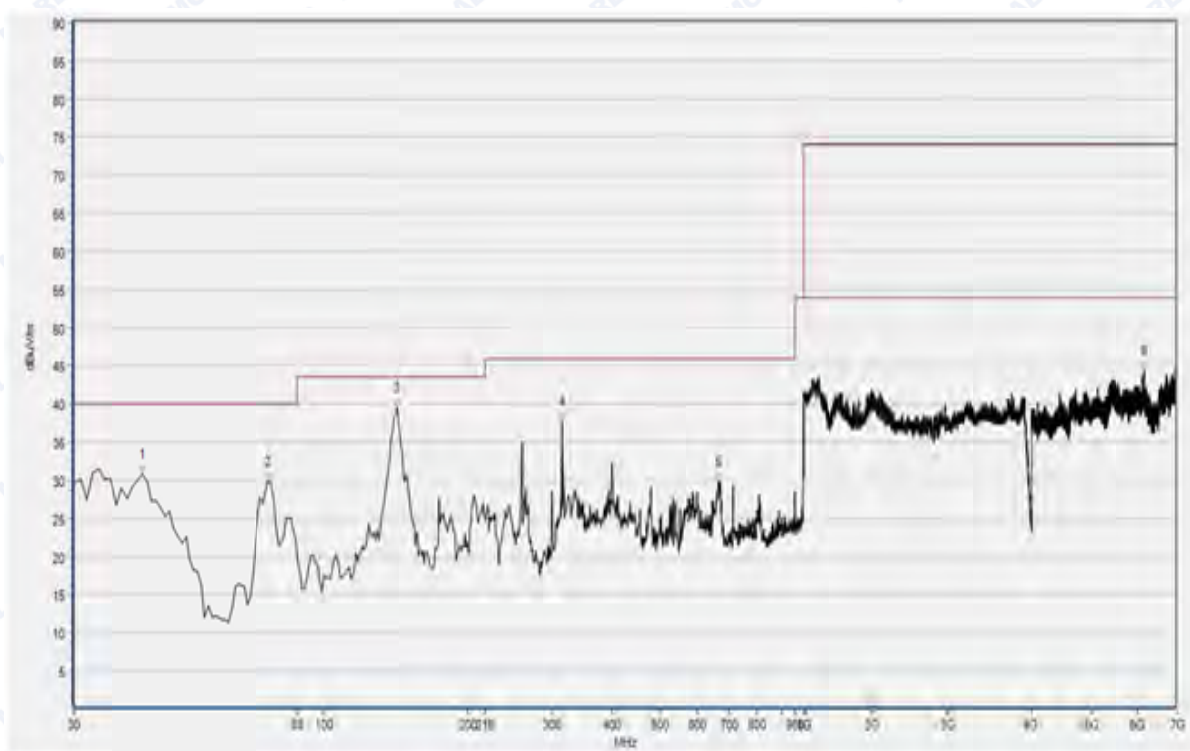
(Plot A: 30MHz – 7GHz, Test Antenna Vertical)
