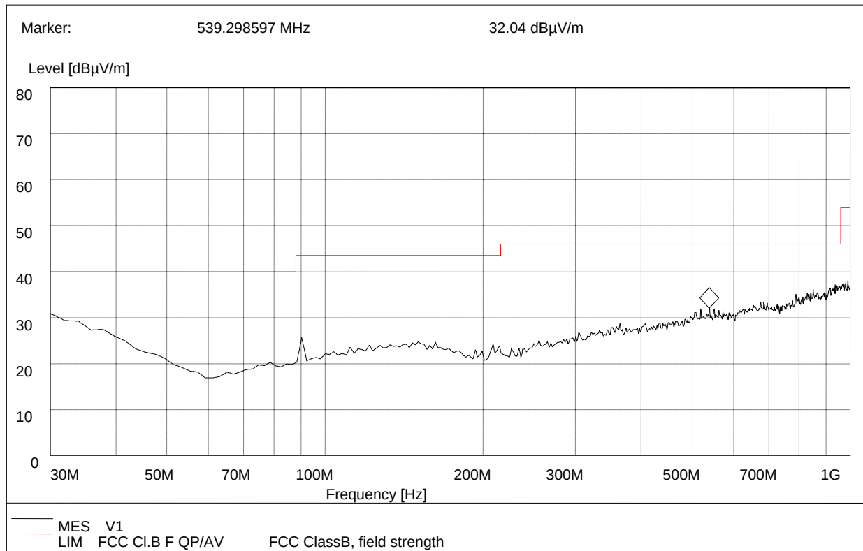
A. (Plot A: Test Antenna Vertical 30M - 1G)
