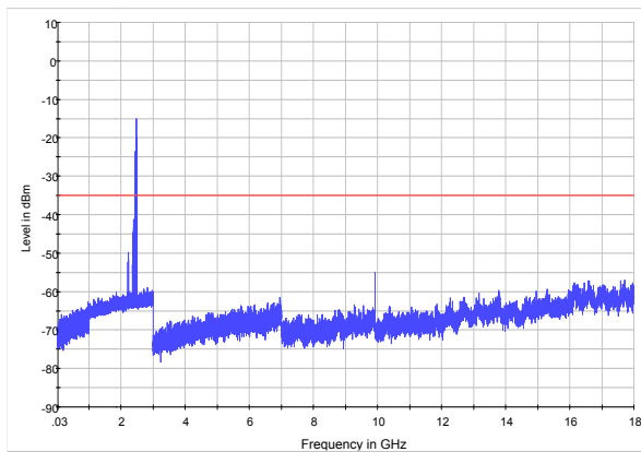
GFSK-CH78 30MHz to 18GHz
