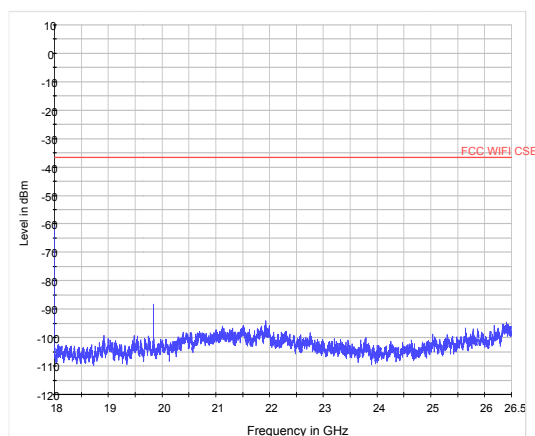
EDR-CH78 18GHz to 26.5GHz
