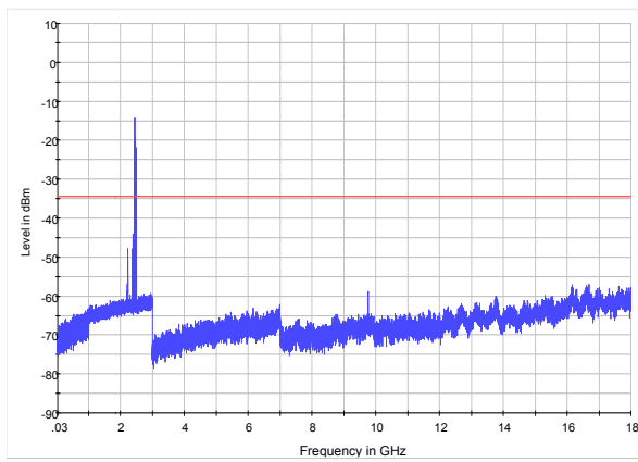
GFSK-CH78 30MHz to 18GHz
