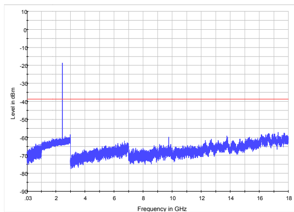
EDR-CH78 30MHz to 18GHz
