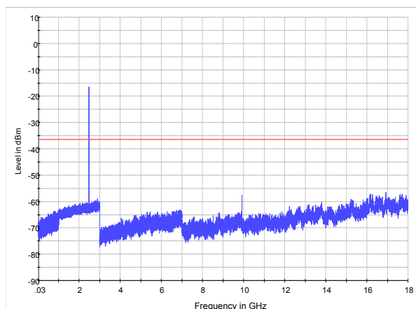
EDR-CH78 30MHz to 18GHz
