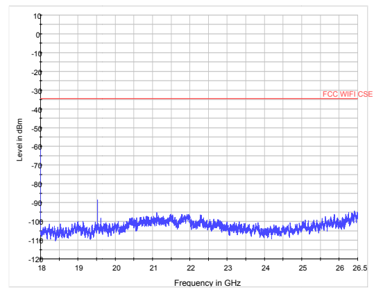
GFSK-CH78 18GHz to 26.5GHz
