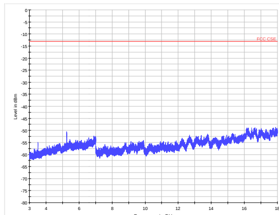
WCDMA Band IV CH-High 3GHz ~18GHz
