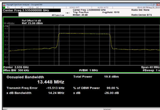
FDD07_MidRange_20_2535_Q16
