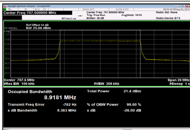
FDD12_MidRange_10_707.5_Q16
