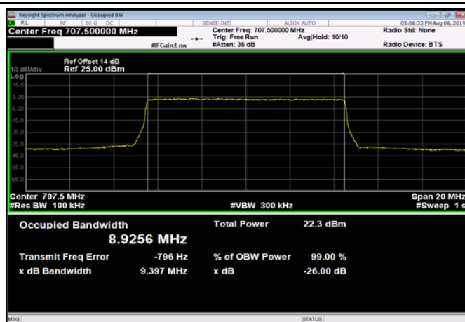
FDD12_MidRange_10MHz_707.5MHz_QPSK
