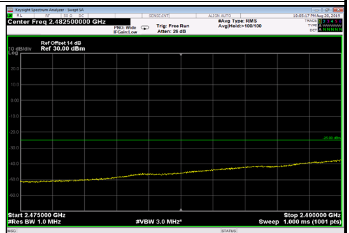
FDD07_15MHz_2507.5_Q16_fullRB_ExtraBands_Range_2475~2490
