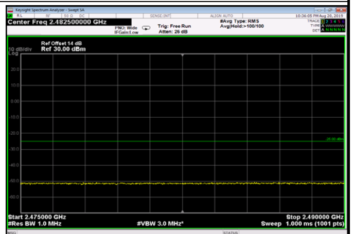
FDD07_20MHz_2560_QPSK_OneRB_low _ExtraBands_Range_2475~2490
