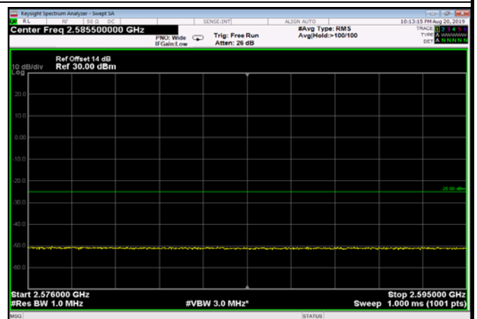
FDD07_20MHz_2510_Q16_fullIRB_ExtraBand s_Range_2576~2595
