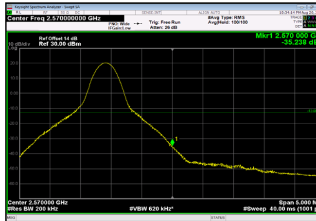
FDD07_20MHz_2560_Q16_OneRB_high _ExtraBands_Range_2570~2575
