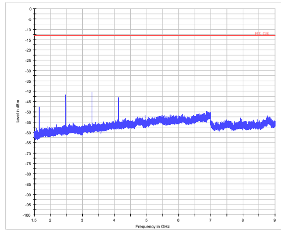
LTE Band 5 10MHz CH-Middle 1.5GHz~9GHz
