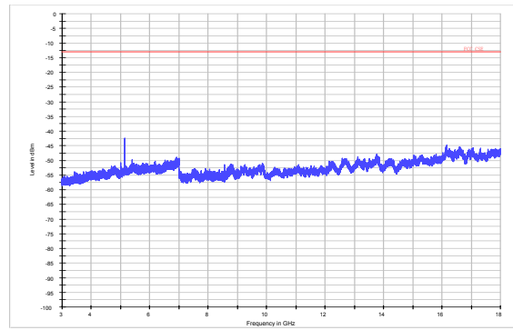
LTE Band 4 10MHz CH-Middle 3GHz~18GHz
