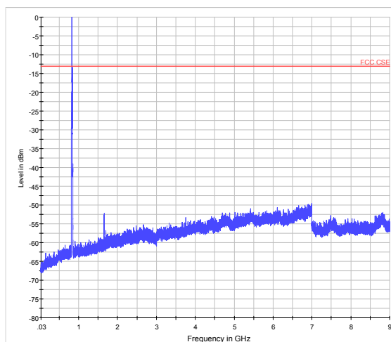
WCDMA Band V CH-Middle 30MHz ~ 9GHz
