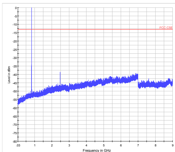
GSM 850 CH-Middle 30MHz ~ 9GHz
