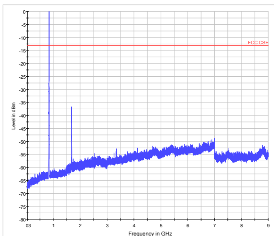
WCDMA Band V CH-Middle 30MHz ~ 9GHz
