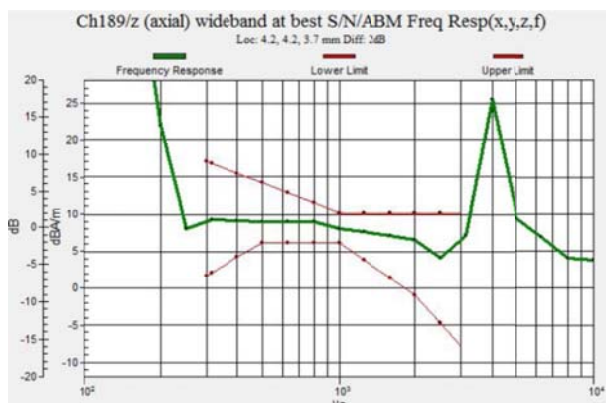
Fig 7.1 GSM850 Ch189
