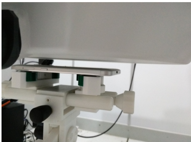
Photo 9: Edge B(10mm)
