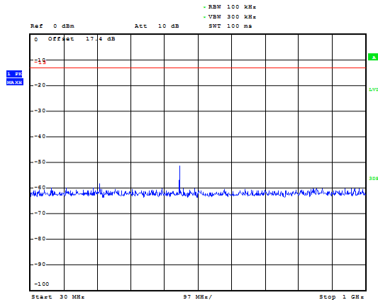
GSM 1900 CH-Middle 30MHz~1GHz
