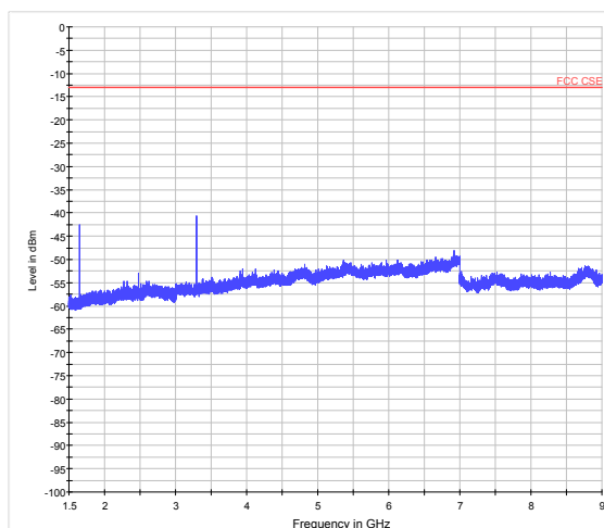
LTE Band 5 10MHz CH-Middle 1.5GHz~9GHz
