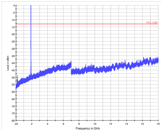
GSM 1900 CH-High 30MHz~18GHz
