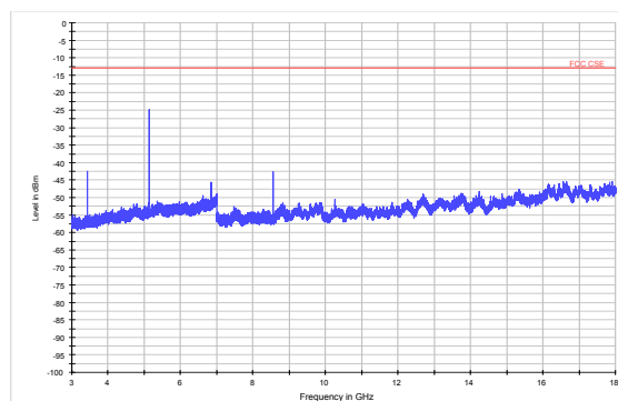
LTE Band 4 5MHz CH-Middle 3GHz~18GHz
