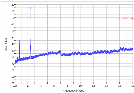
802.11b CH12 30MHz to 18GHz
