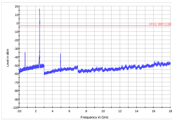
802.11b CH13 30MHz to 18GHz
