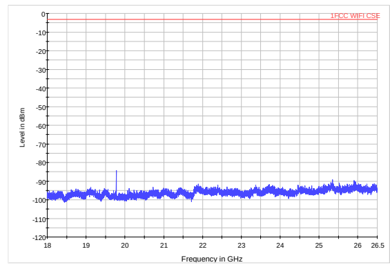
802.11b CH13 18GHz to 26.5GHz
