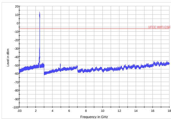
802.11n (HT20) CH13 30MHz to 18GHz
