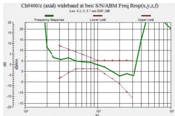
Fig 9.4 WCDMA Band II Ch9400
