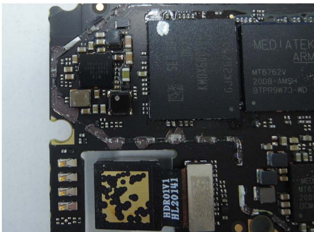
IC Details 8
