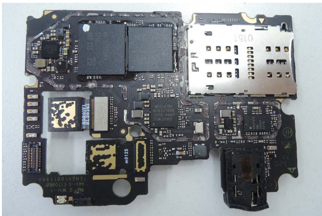
IC Details 6
