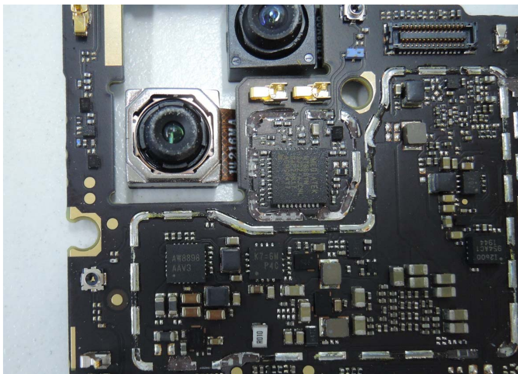
IC Details 3
